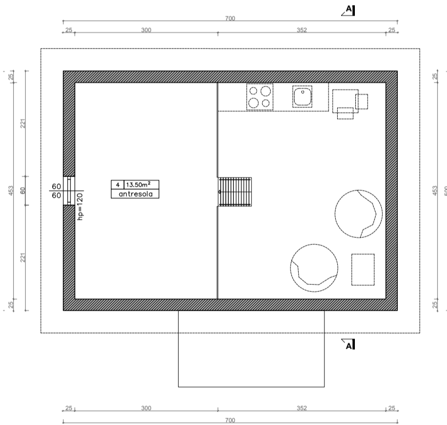
RZUT ANTRESOLI
