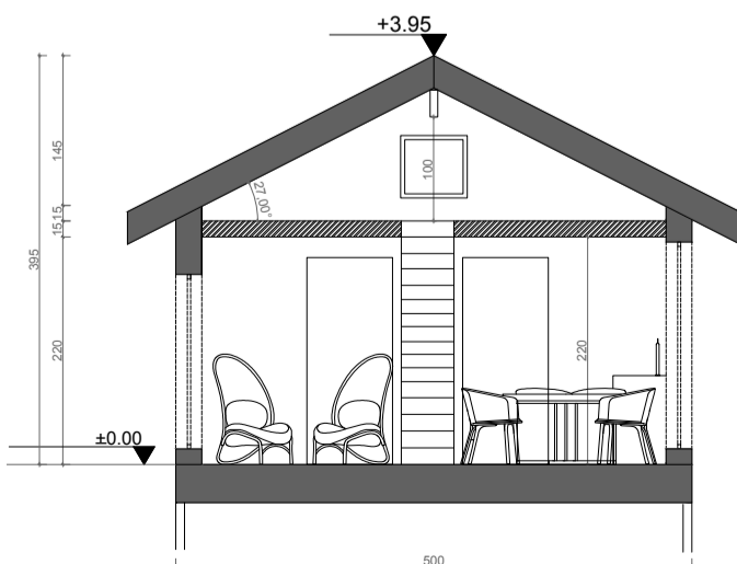
PRZEKRÓJ A-A
