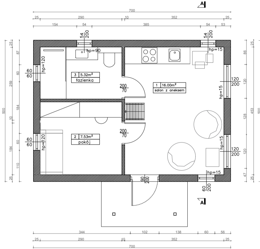
RZUT PARTERU
